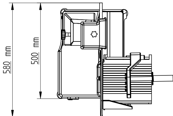
Boven aanzicht
